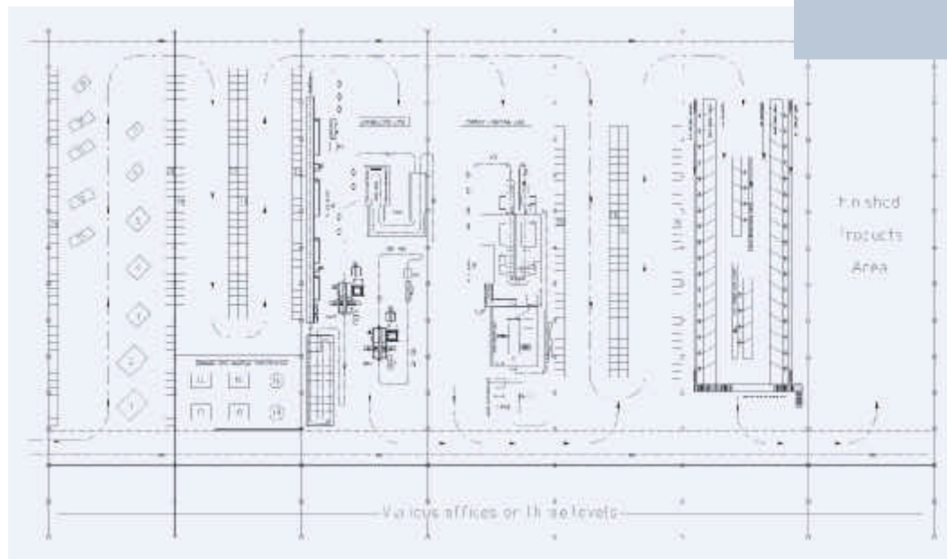
Lay-out di un impianto completo per la produzione di cucine. Lay-out of complete plant for cookers production.
